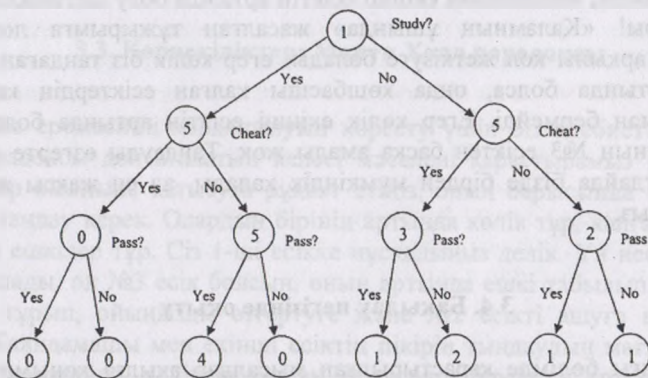
3.1-сурет. Бақылау ағашы
