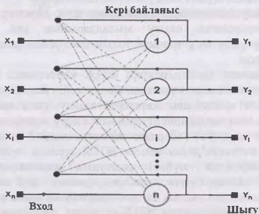
4.11-сурет. Хопфилд желісінің құрылымдық схемасы
